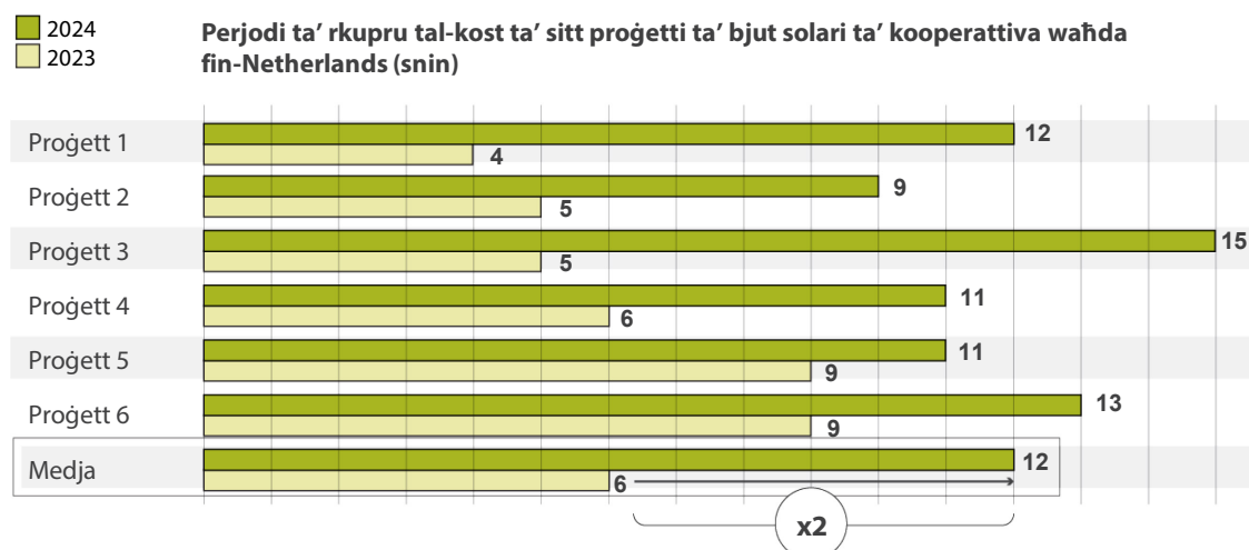
Figura 13 | Il-perjodi ta' rkupru tal-kost jallinjaw mal-aspettattivi tal-Istrategija dwar l-Energija Solari, iżda jvarjaw skont il-prezzijiet tal-enerġija u l-kalkolu tal-primjum “feed-in”
