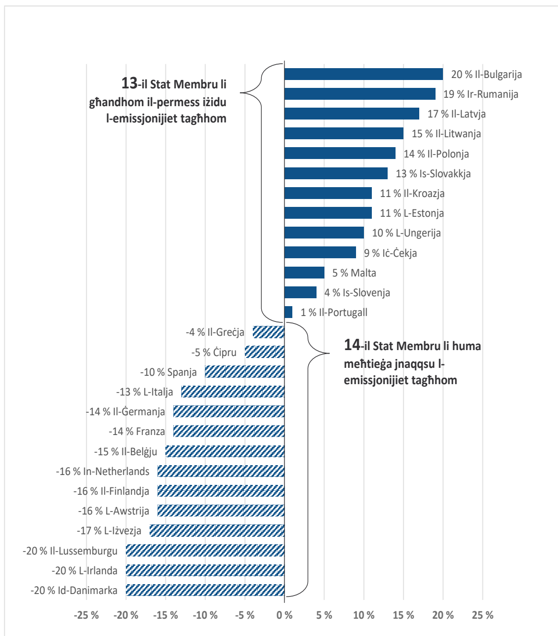
Figura 5 – Miri nazzjonali għall-2020 skont il-legizlazzjoni dwar il-kondiviżjoni tal-isforzi, meta mqabbla mal-emissjonijiet tal-2005
