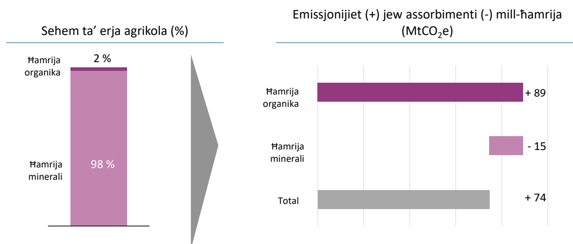
Figura 21 – Filwaqt li fl-2018 il-ħamrija organika kienet tirrappreżenta 2 % tal-ħamrija tal-UE, hija responsabbli għall-biċċa l-kbira mill-emissjonijiet ta' gassijiet serra li ġejjin mill-użu tal-art
