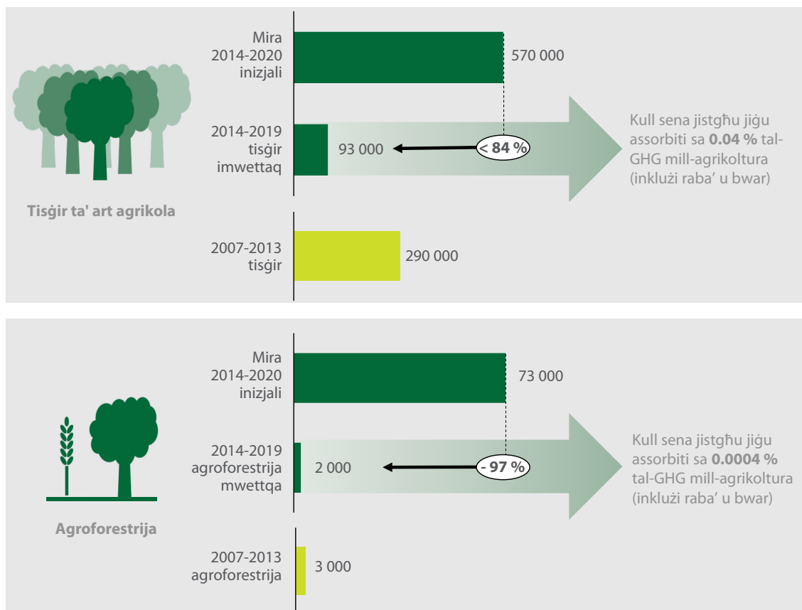
Figura 23 – Tisgħir u agroforestrija fil-perjodu 2014-2020 u fil-perjodu 2007-2013 (ettari)
