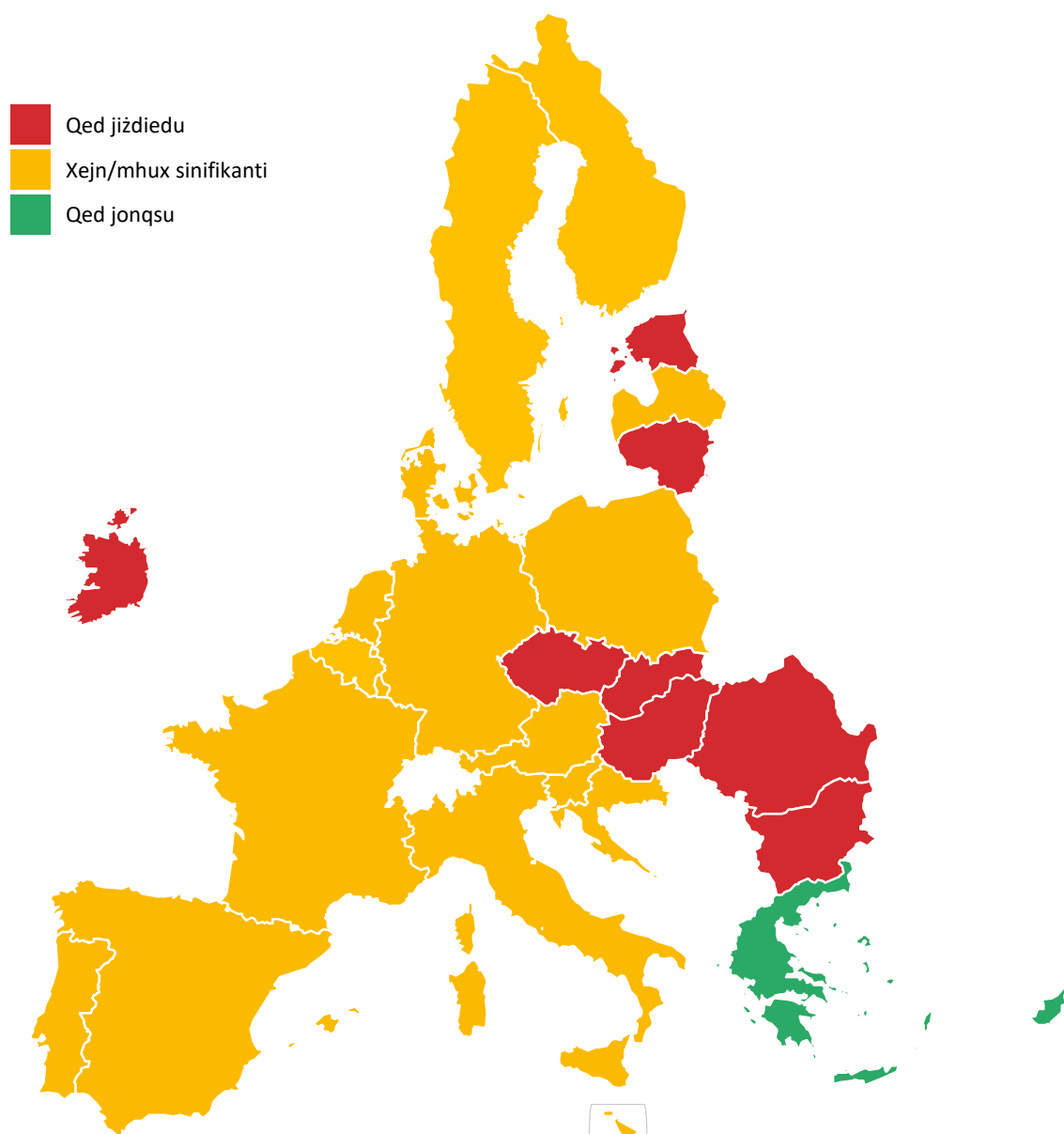
Figura 15 – Xejriet tal-emissjonijiet min-nutrijenti tal-ħamrija għall-perjodu 2010-2018
