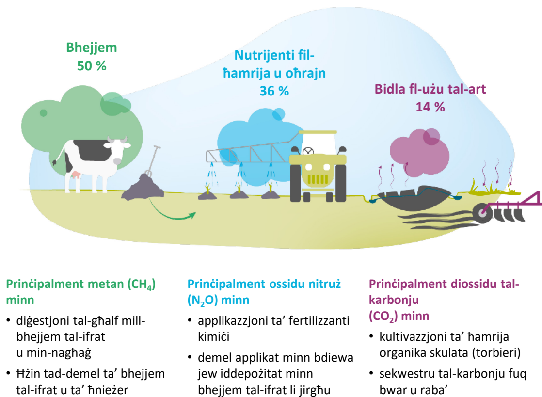
Figura 2 – Sorsi ewlenin tal-emissjonijiet ta' gassijiet serra (f'CO 2 e)
