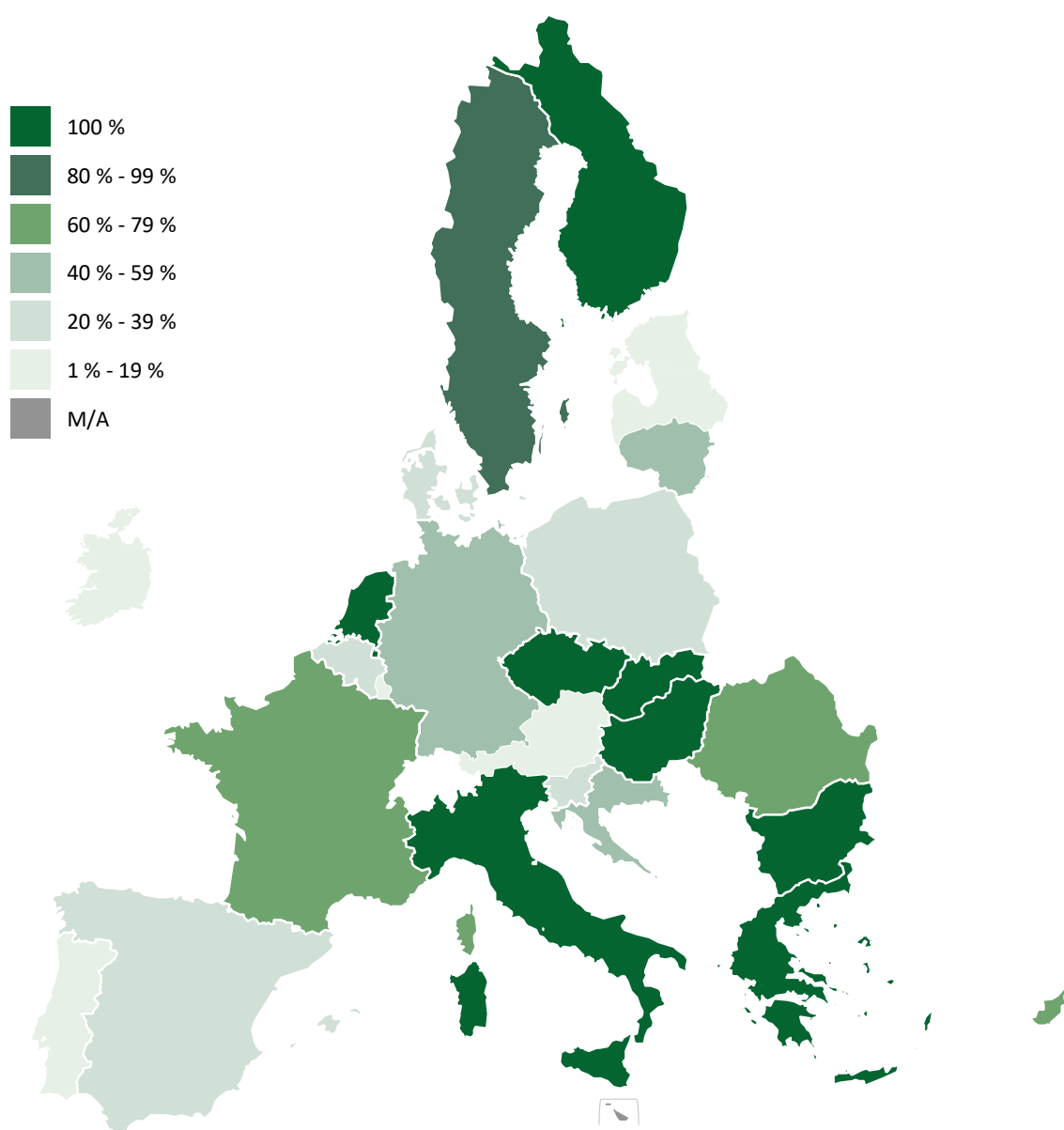
Figura 22 – Sehem ta' bwar permanenti iddeżinjati bħala ambjentalment sensittivi fi hdan Natura 2000 fl-UE
