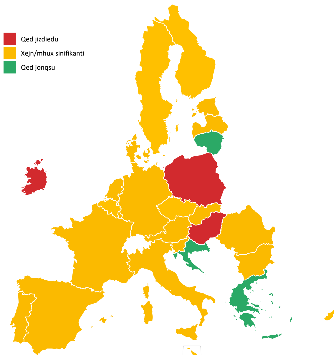
Figura 10 – Xejriet tal-emissjonijiet mill-bhejjem għall-perjodu 2010-2018
