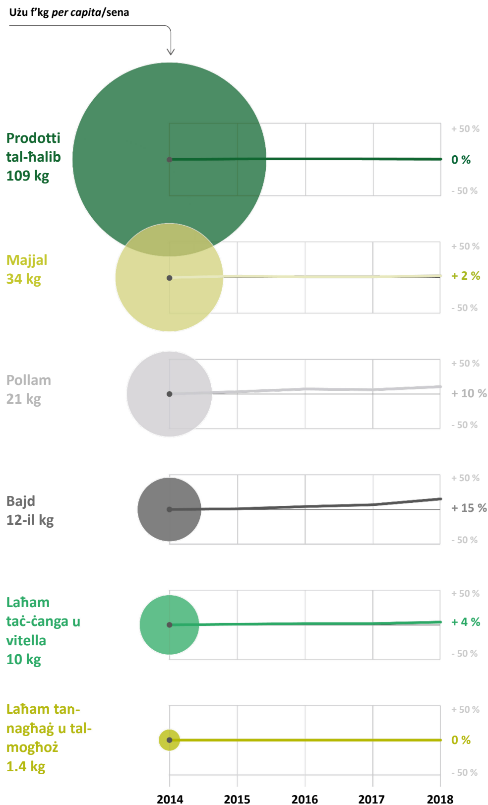
Figura 11 – Mhuwiex qed jonqos il-konsum annwali per capita ta' prodotti li ġejjin mill-annimali fl-UE
