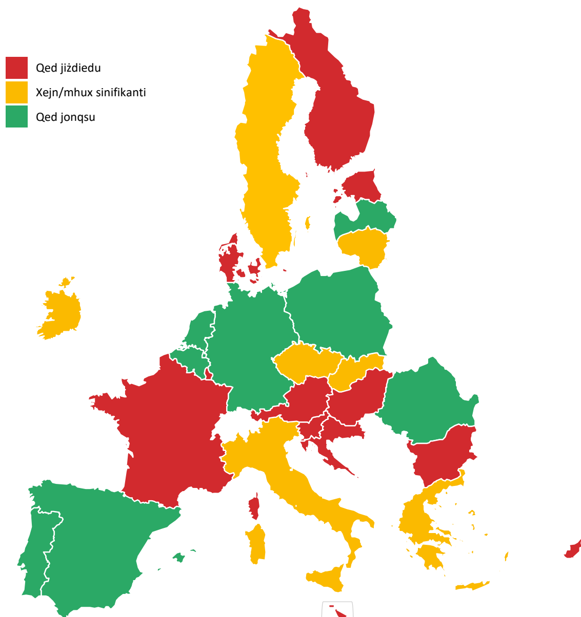
Figura 18 – Xejriet tal-emissjonijiet mill-użu tal-art għall-perjodu 2010-2018
