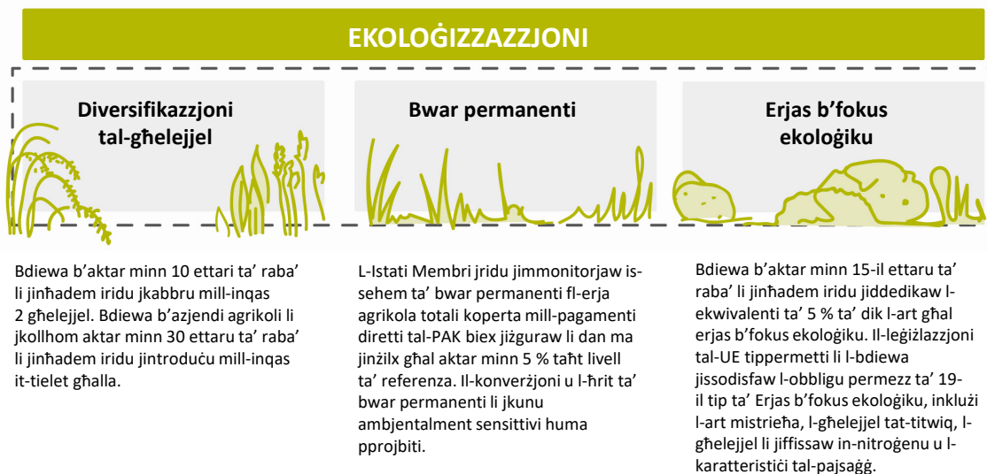
Figura 25 – Arkitettura ta' ekoloġizzazzjoni
