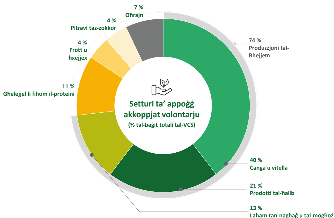
Figura 12 – Sehem settorjali tal-appoġġ tal-VCS
