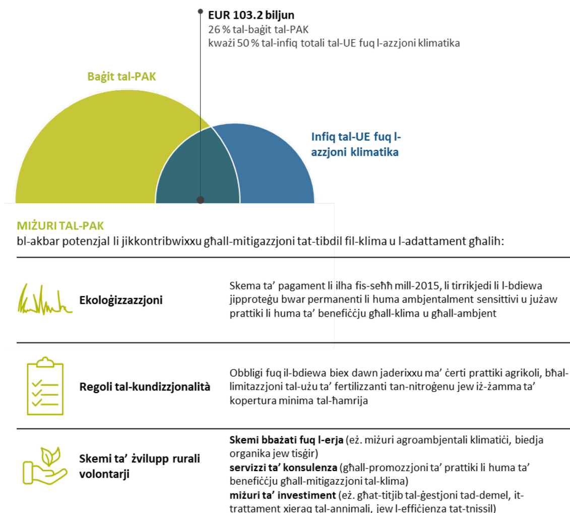
Figura 7 – Miżuri ewlenin tal-PAK użati għall-azzjoni klimatika skont il-Kummissjoni, il-perjodu 2014-2020
