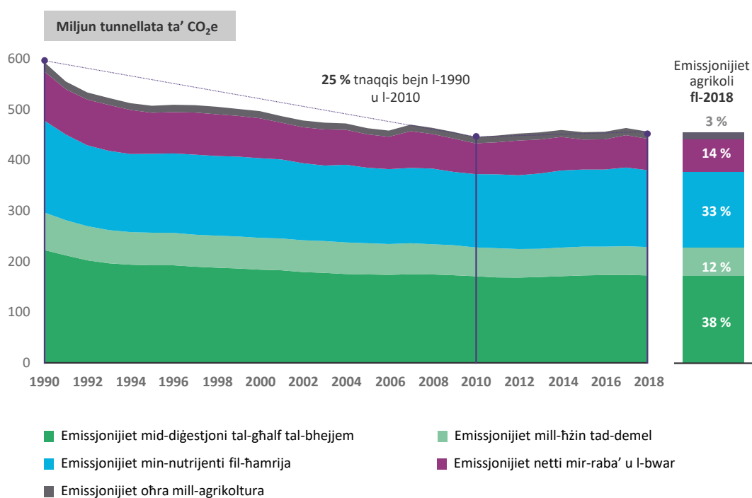
Figura 3 – Emissjonijiet netti ta' gassijiet serra mill-agrikoltura għall-EU-27 mill-1990 'il hawn
