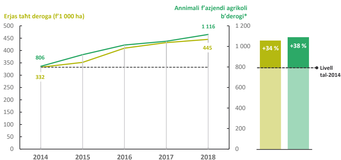
Figura 16 – Evoluzzjoni tal-erjas Irlandiżi taħt deroga mid-Direttiva dwar in-Nitrati u l-għadd assoċjat ta' annimali
