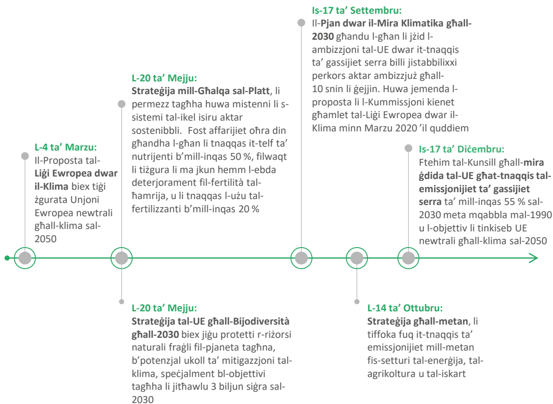
Figura 8 – Strateġiji, proposti u ftehimiet tal-UE rigward it-tibdil fil-klima u l-agrikoltura ppubblikati fl-2020
