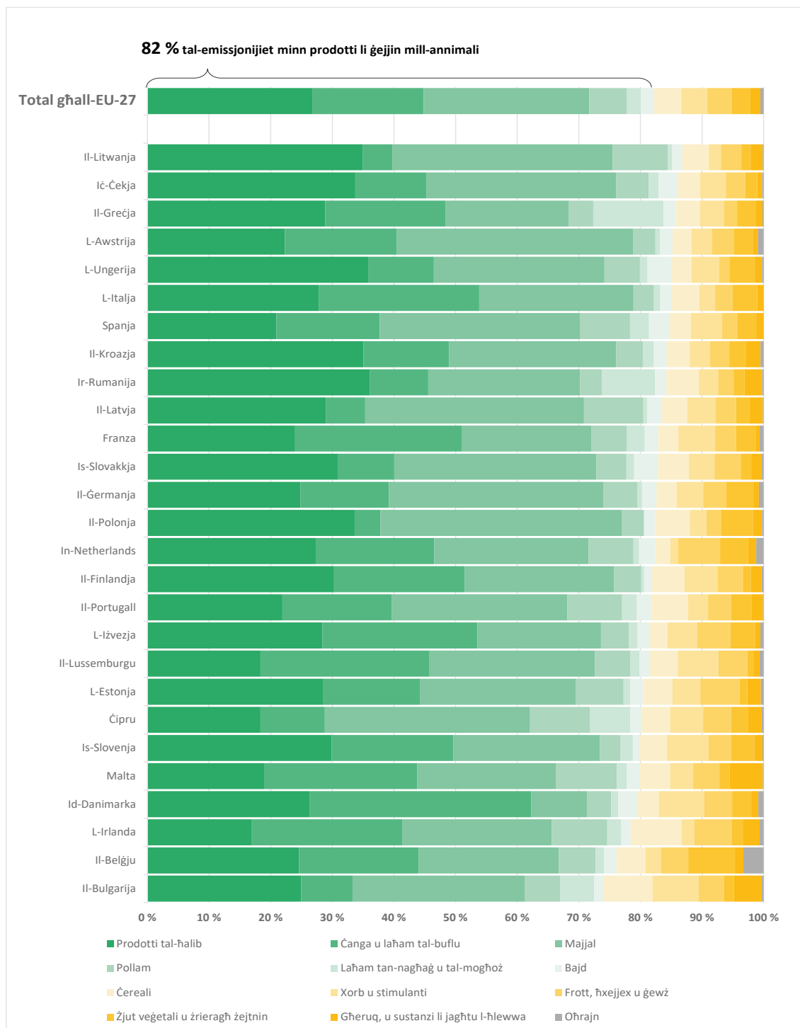
Figura 13 – Impronta tal-karbonju li titħalla mill-ikel fid-dieta tal-UE
