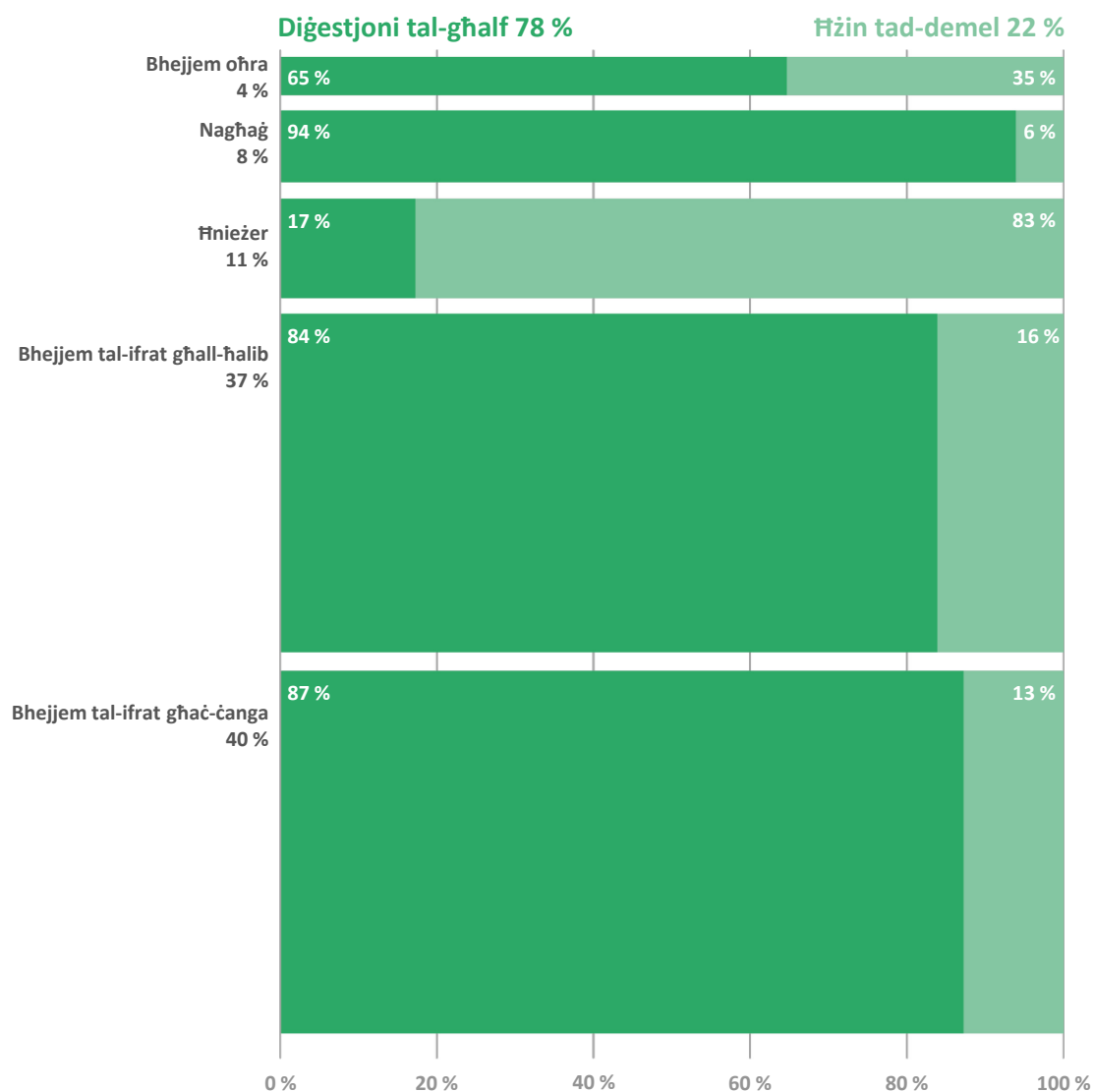
Figura 9 – Sorsi ta' emissjonijiet mill-bhejjem fl-2018
