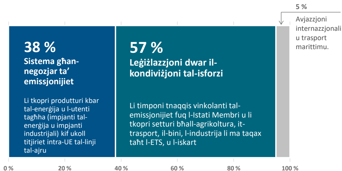
Figura 4 – Qafas tal-UE għall-mitigazzjoni tat-tibdil fil-klima fl-2018
