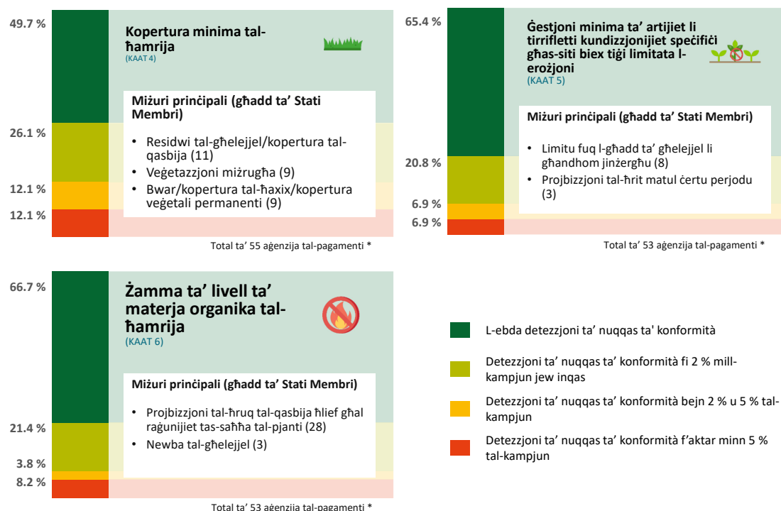
Figura 24 – Percentwal ta' aġenziji tal-pagamenti għal kull livell ta' ksur tal-kundizzjonalità li nstab, għal tliet regoli tal-kundizzjonalità li huma ta' benefiċċju għall-klima (medja għall-perjodu 2015-2017)
