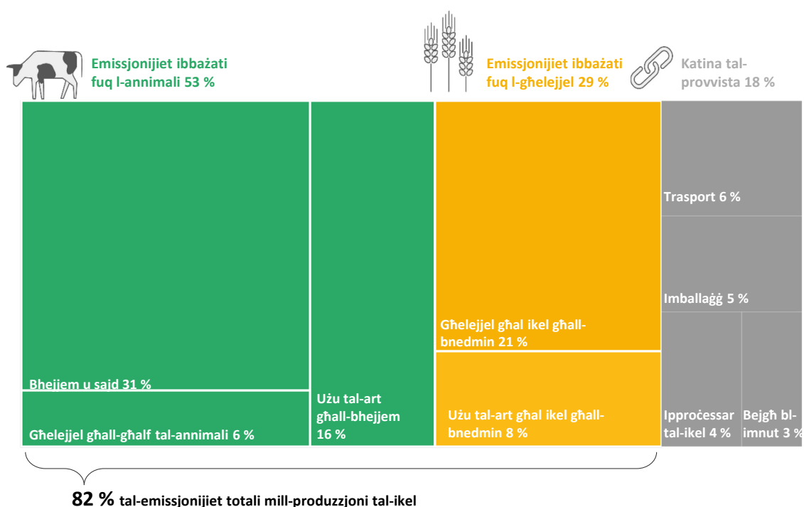
Figura 1 – Emissjonijiet globali ta' gassijiet serra mill-produzzjoni tal-ikel
