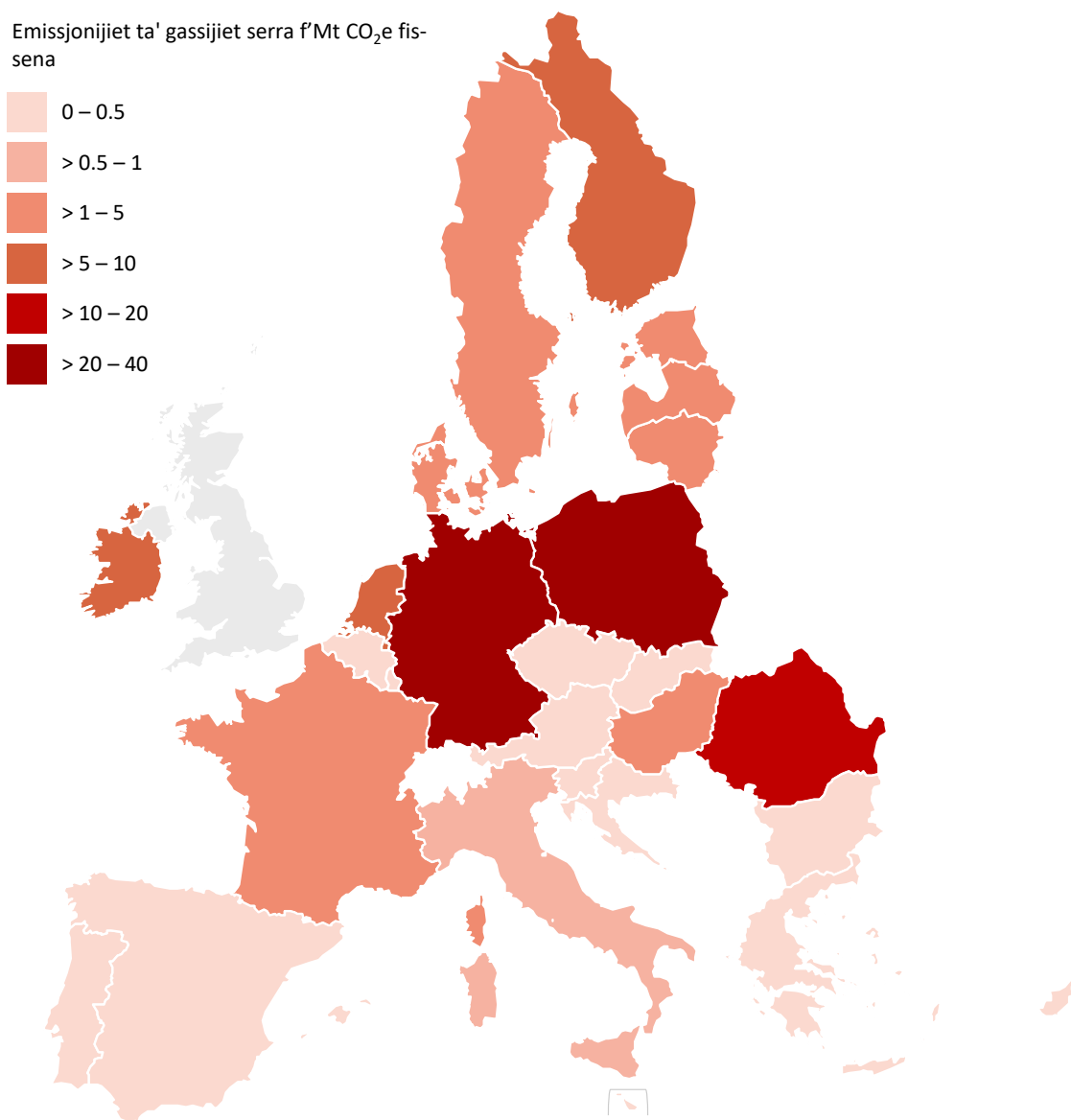
Figura 20 – Emissjonijiet ta' gassijiet serra minn ħamrija organika kkultivata
