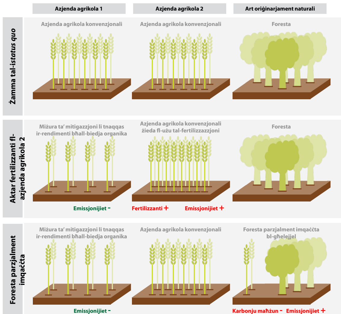
Figura 17 – Prattiki li jnaqqsu r-rendimenti jistgħu jittrasferixxu l-emissjonijiet ta' gassijiet serra lejn azjendi agrikoli oħra
