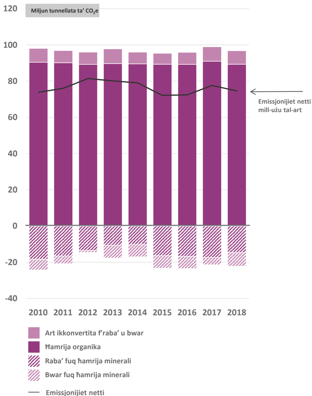
Figura 19 – Emissjonijiet u assorbimenti minn ħamrija organika u minerali
