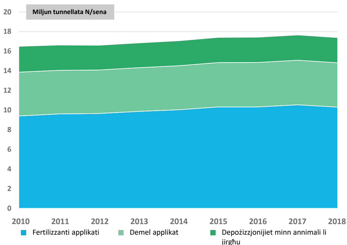
Figura 14 – Applikazzjoni ta' fertilizzanti kimiċi u ta' demel tal-bhejjem
