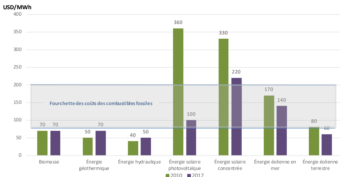
Figure 3 – LCOE global des technologies de production d'électricité à partir de sources renouvelables, 2010-2017 (en dollars des États-Unis/MWh)
